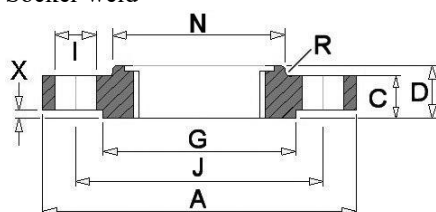
Socker weld
